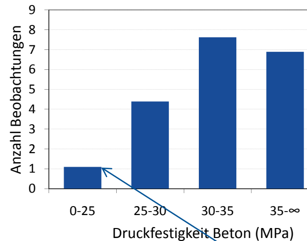
Erwartetes Histogramm
